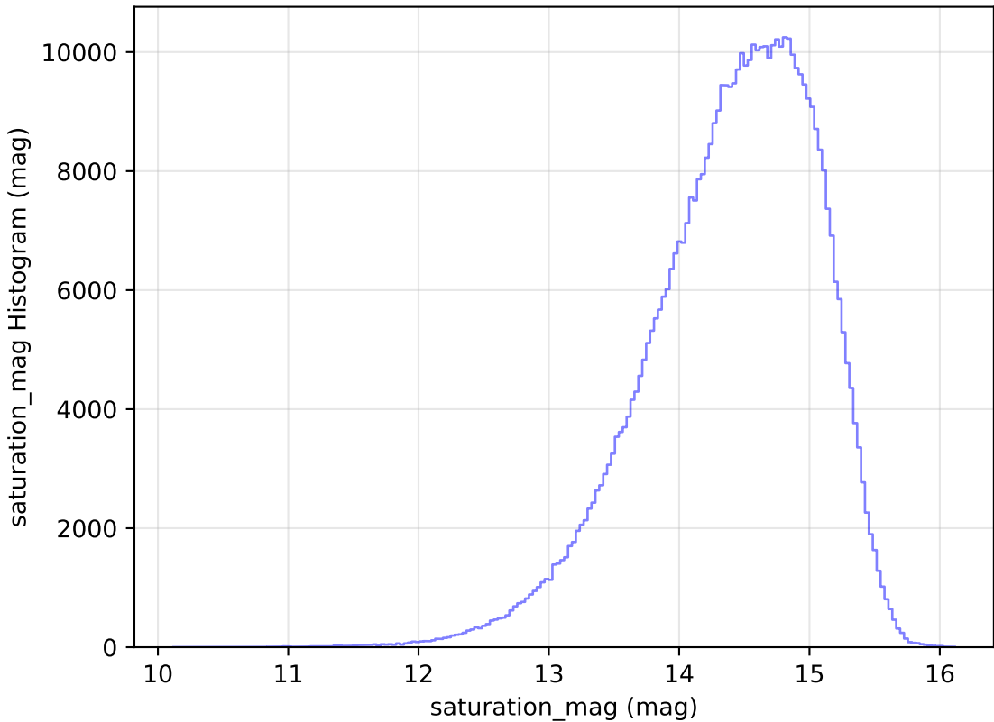
weather_cloudso6v3.4_10yrs WFD i band: saturation_mag Histogram
