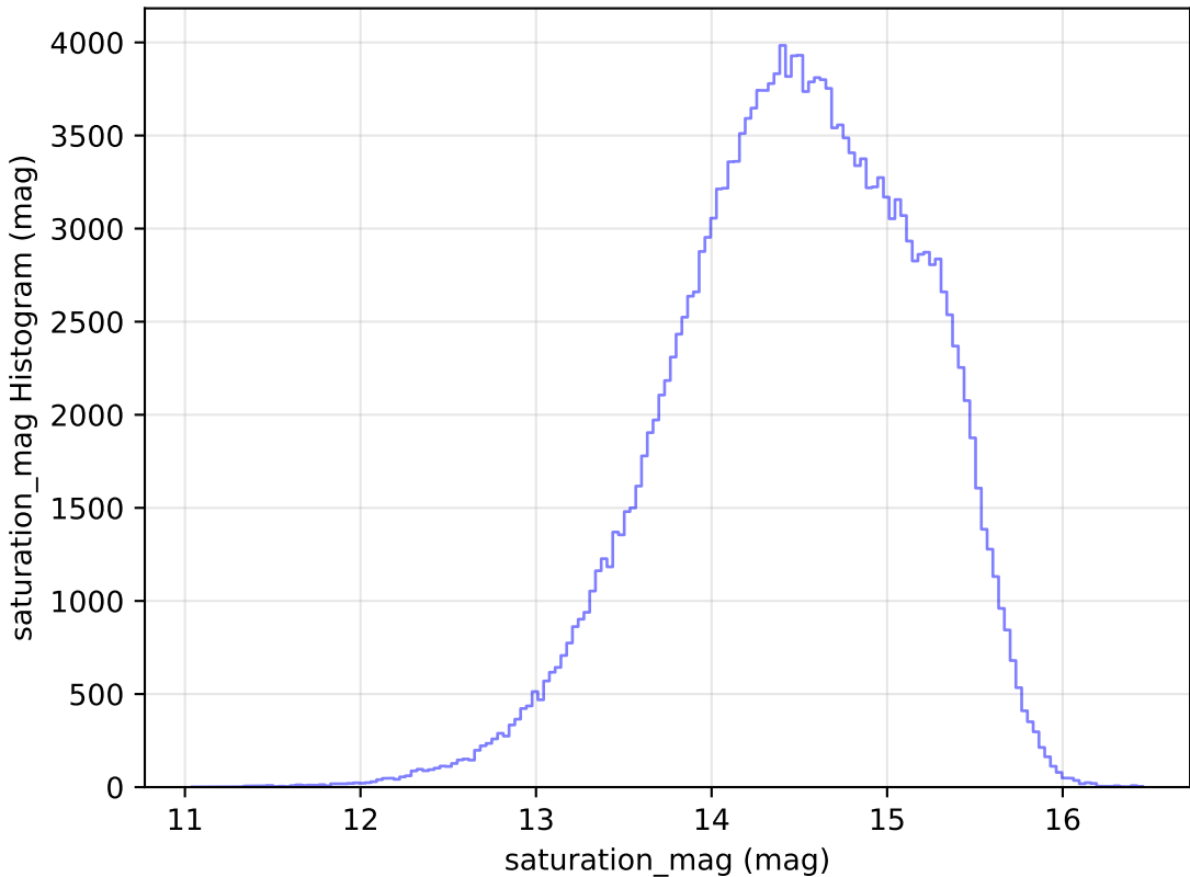
weather_cloudso6v3.4_10yrs WFD g band: saturation_mag Histogram
