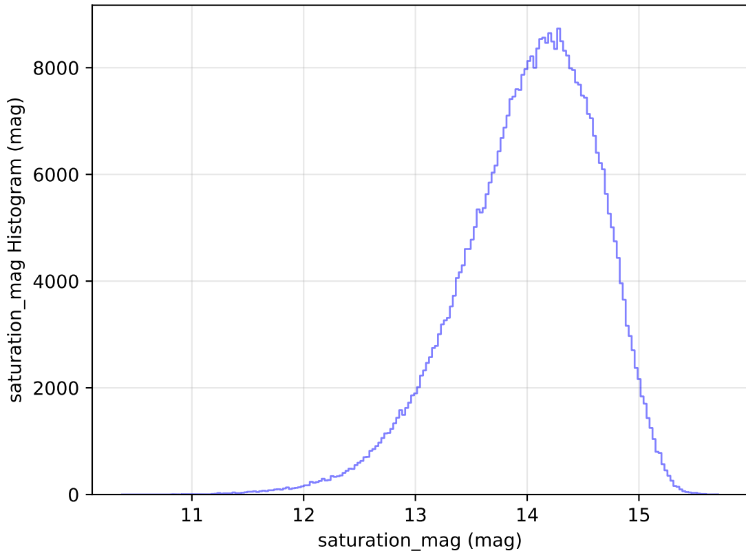
weather_cloudso6v3.4_10yrs All sky z band: saturation_mag Histogram
