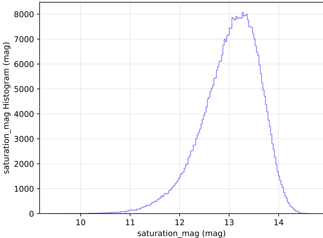
weather_cloudso6v3.4_10yrs All sky y band: saturation_mag Histogram
