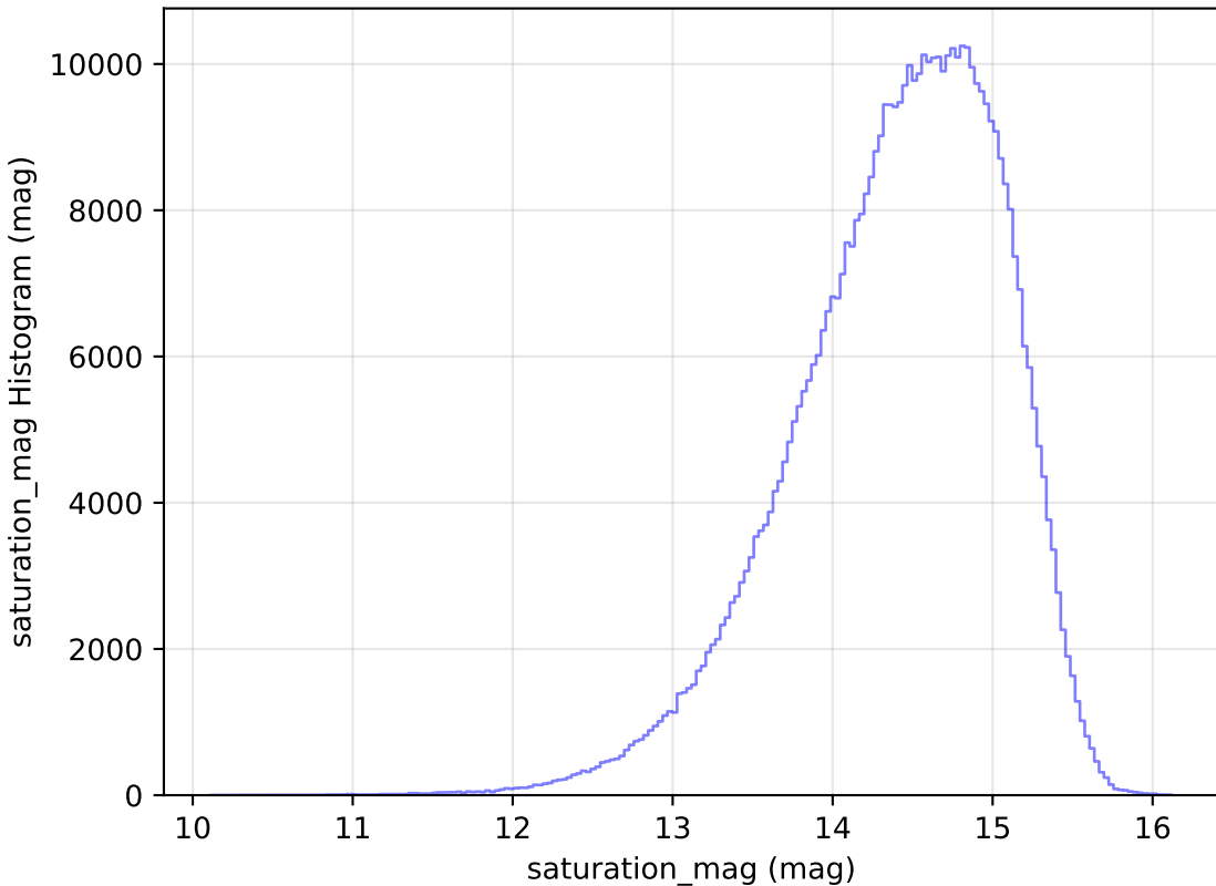
weather_cloudso6v3.4_10yrs All sky i band: saturation_mag Histogram
