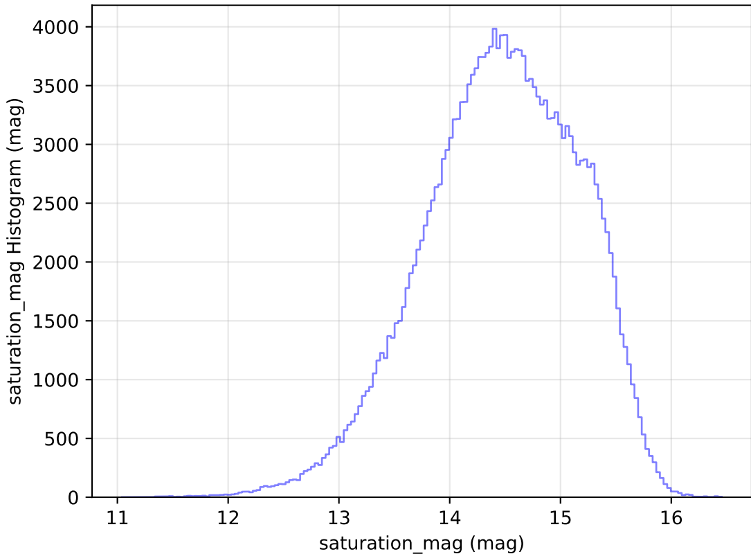
weather_cloudso6v3.4_10yrs All sky g band: saturation_mag Histogram
