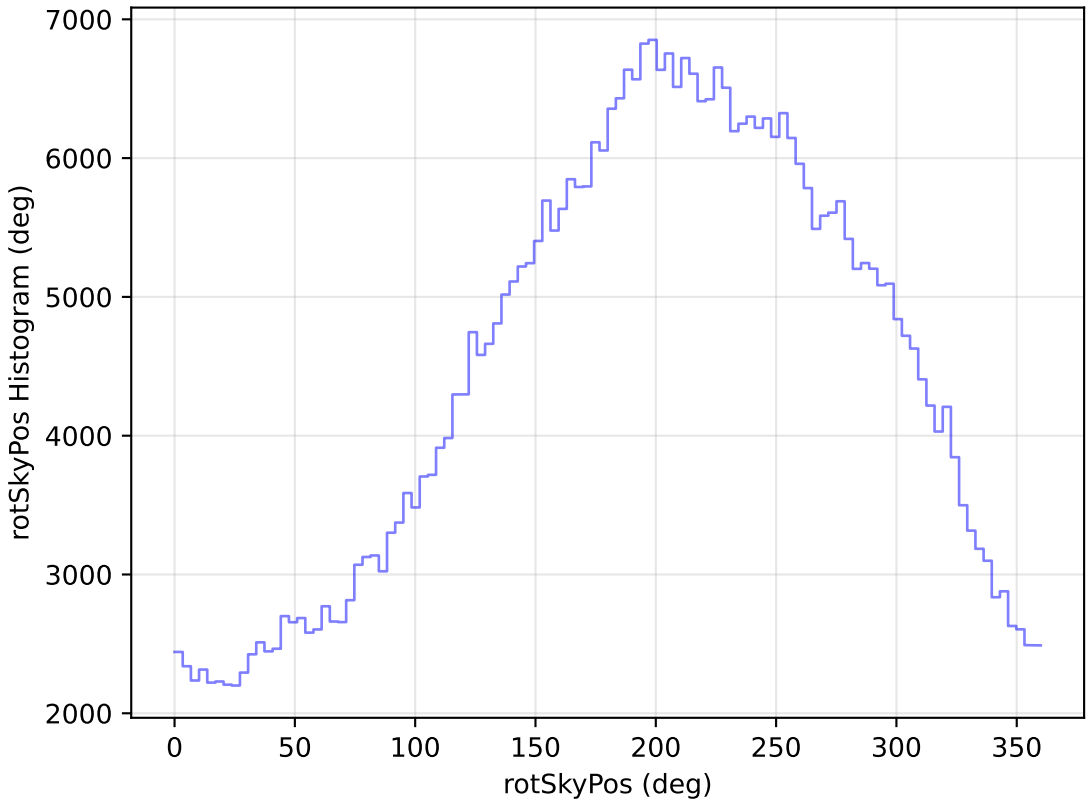
weather_cloudso6v3.4_10yrs WFD z band: rotSkyPos Histogram
