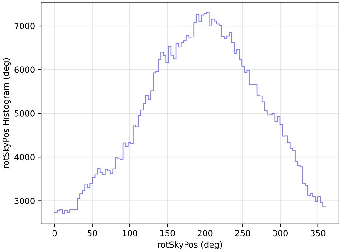
weather_cloudso6v3.4_10yrs WFD r band: rotSkyPos Histogram
