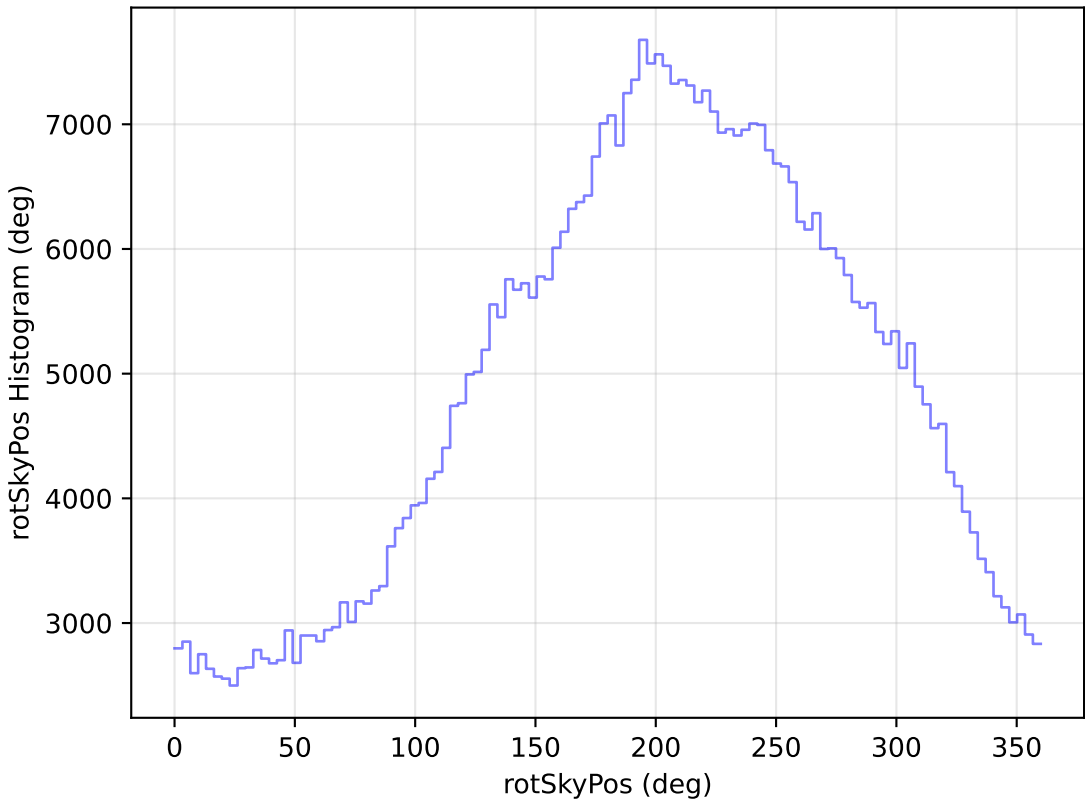
weather_cloudso6v3.4_10yrs WFD i band: rotSkyPos Histogram
