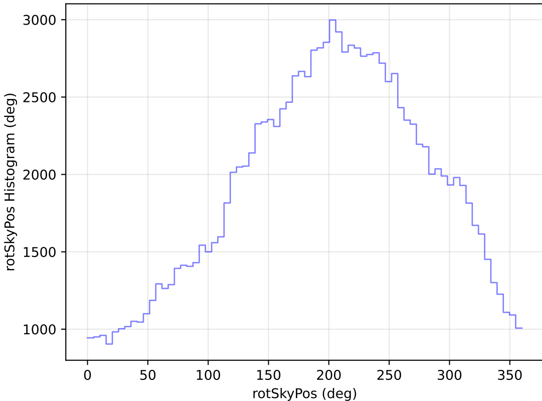
weather_cloudso6v3.4_10yrs All sky u band: rotSkyPos Histogram
