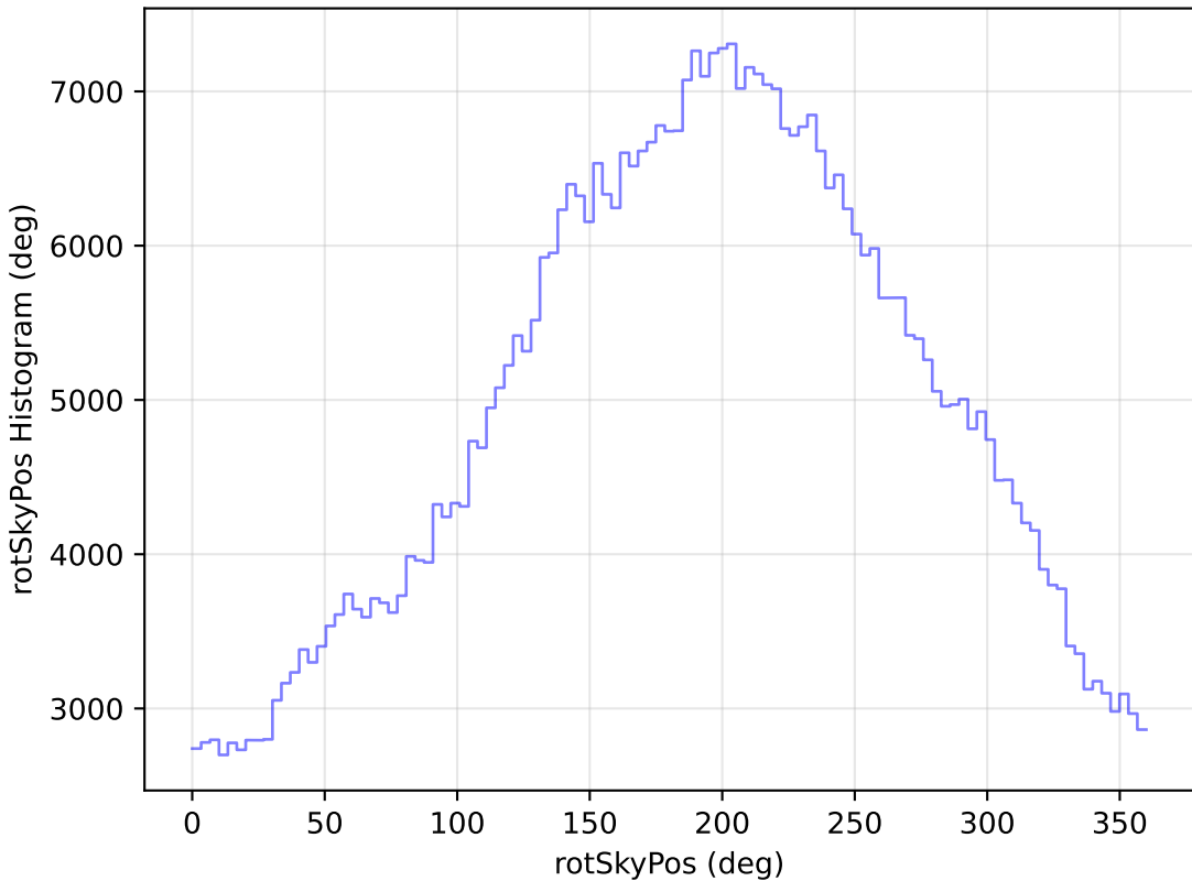
weather_cloudso6v3.4_10yrs All sky r band: rotSkyPos Histogram
