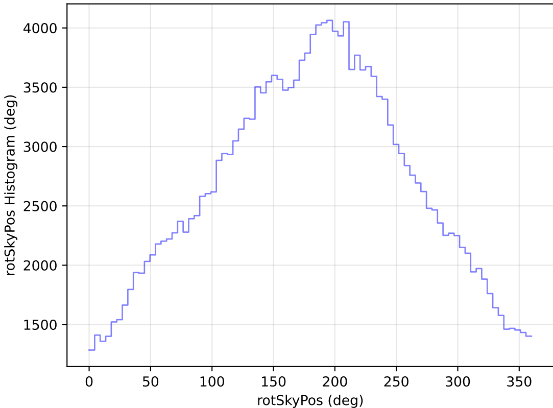
weather_cloudso6v3.4_10yrs All sky g band: rotSkyPos Histogram
