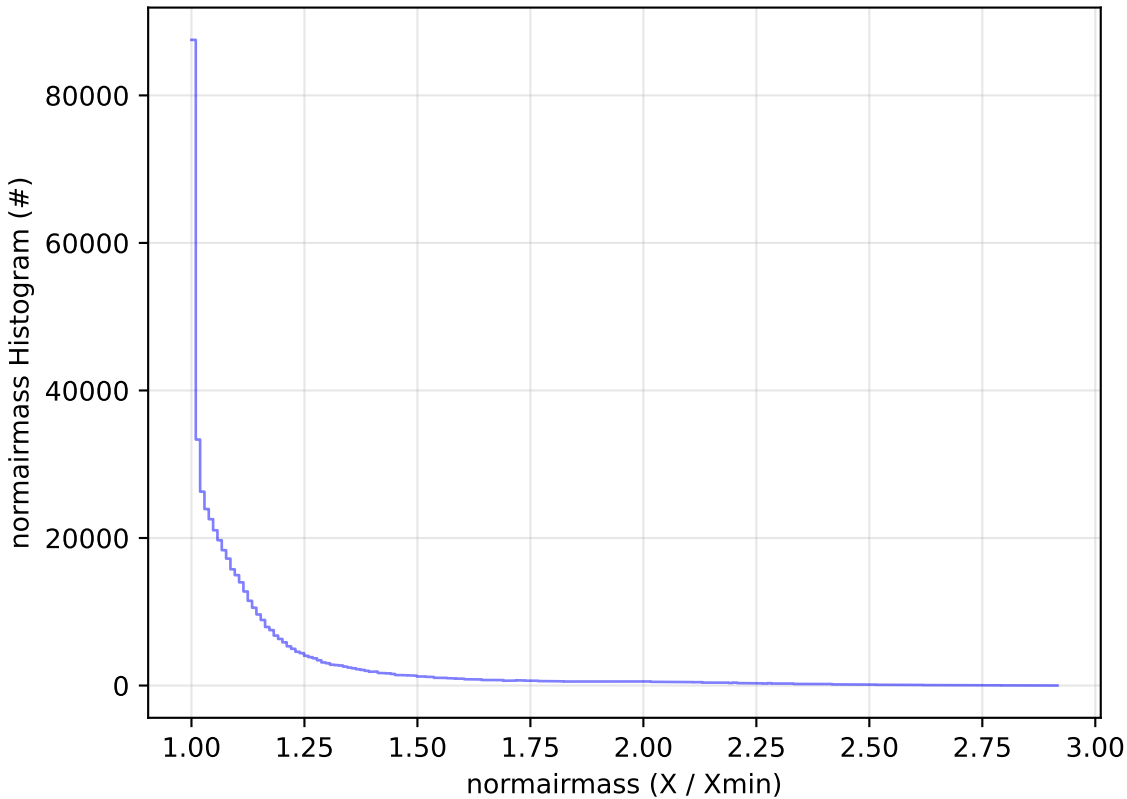
weather_cloudso6v3.4_10yrs WFD i band: normairmass Histogram
