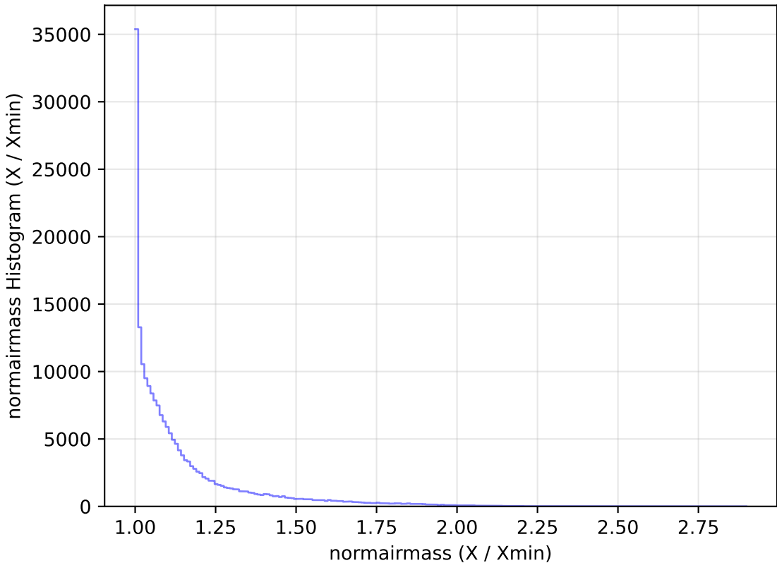
weather_cloudso6v3.4_10yrs WFD g band: normairmass Histogram
