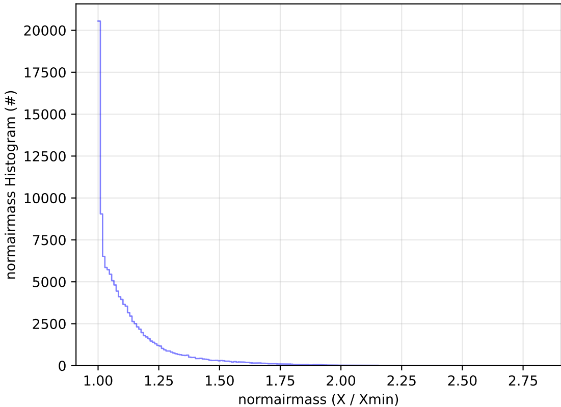
weather_cloudso6v3.4_10yrs All sky u band: normairmass Histogram
