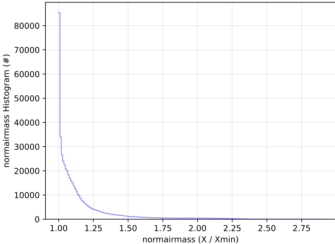
weather_cloudso6v3.4_10yrs All sky r band: normairmass Histogram
