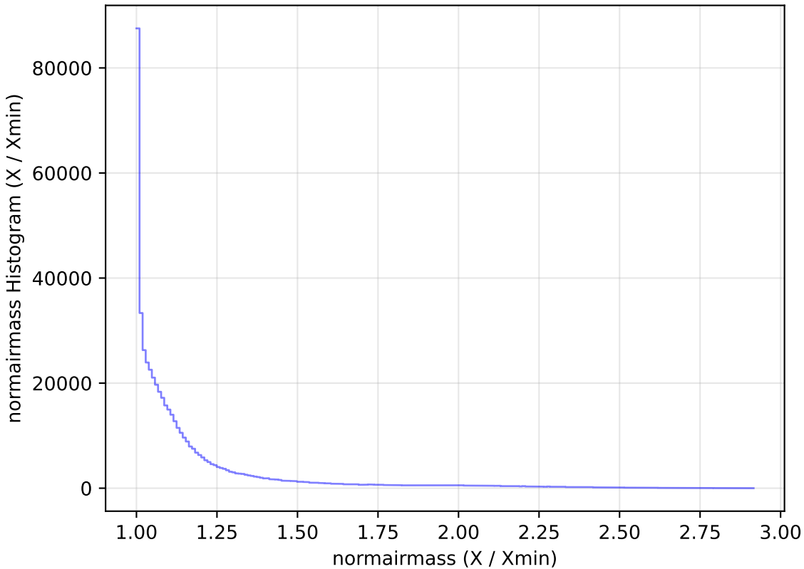
weather_cloudso6v3.4_10yrs All sky i band: normairmass Histogram
