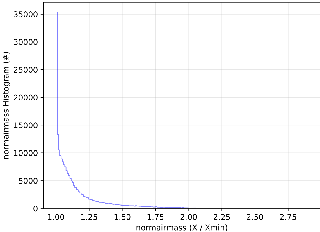
weather_cloudso6v3.4_10yrs All sky g band: normairmass Histogram
