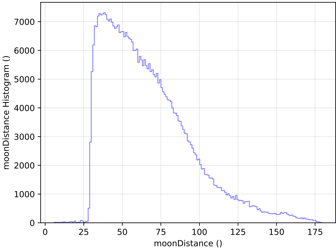
weather_cloudso6v3.4_10yrs WFD y band: moonDistance Histogram
