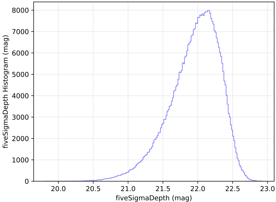
weather_cloudso6v3.4_10yrs WFD y band: fiveSigmaDepth Histogram
