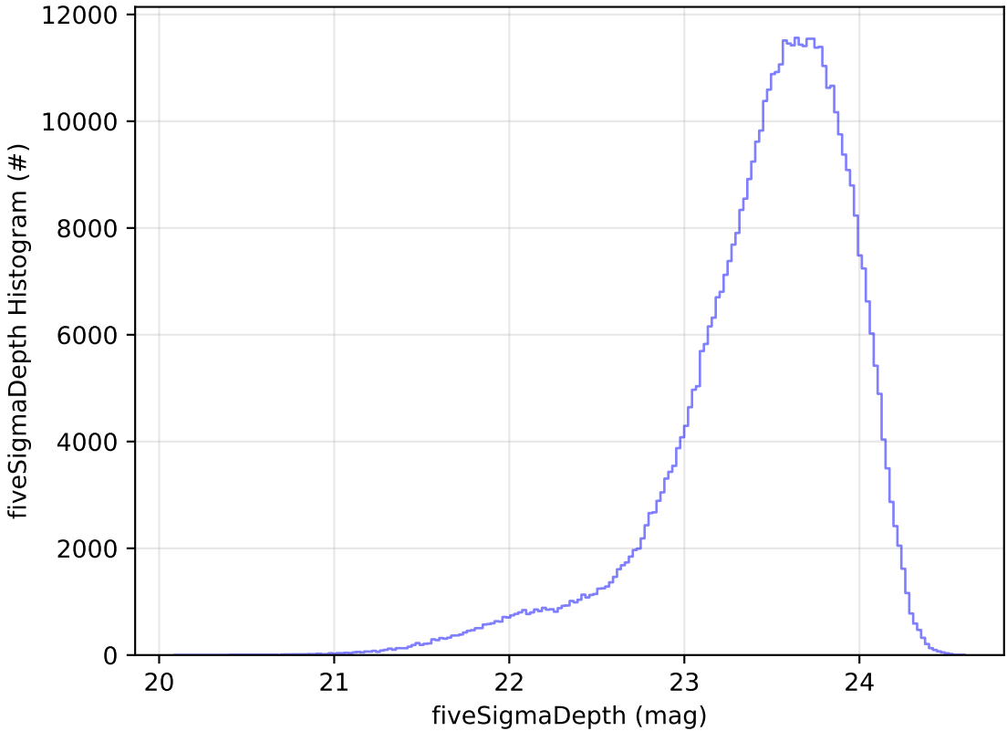
weather_cloudso6v3.4_10yrs WFD i band: fiveSigmaDepth Histogram
