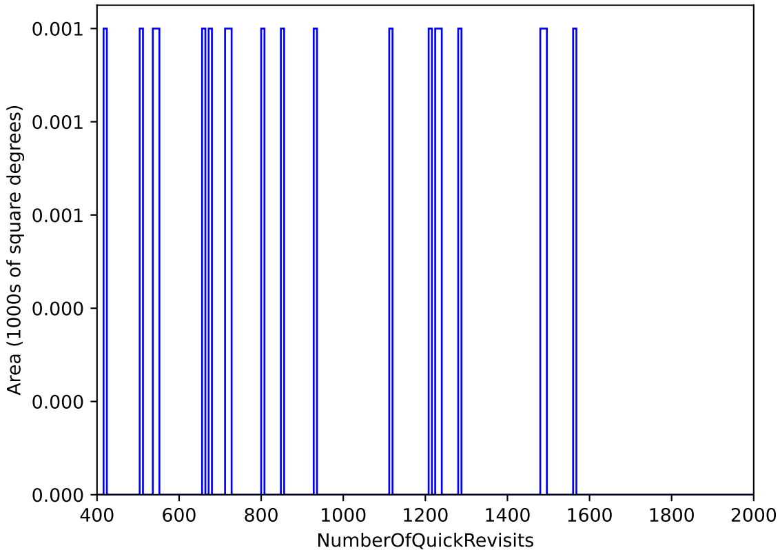
weather_cloudso6v3.4_10yrs WFD: NumberOfQuickRevisits
