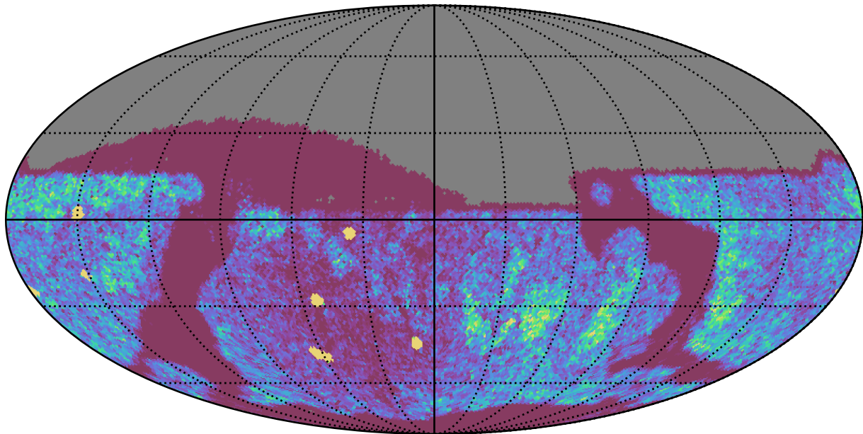
weather_cloudso6v3.4_10yrs Yr 1 z band: NVisits
