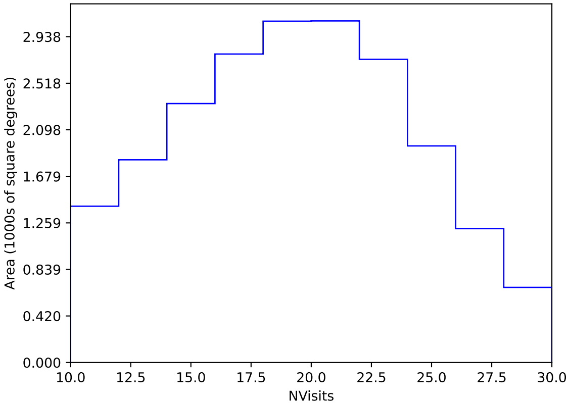
weather_cloudso6v3.4_10yrs Yr 1 y band: NVisits
