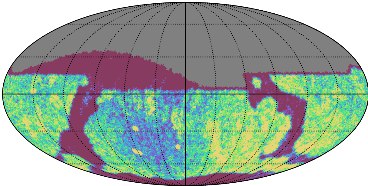
weather_cloudso6v3.4_10yrs Yr 1 i band: NVisits
