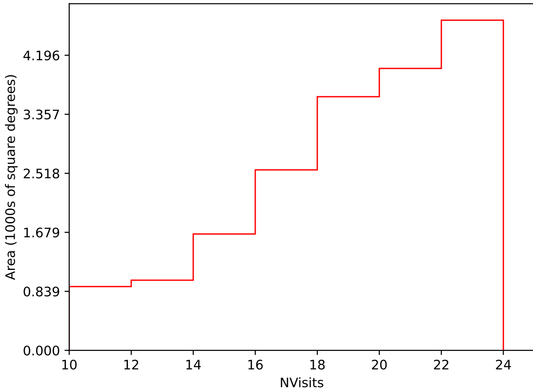
weather_cloudso6v3.4_10yrs Yr 1 i band: NVisits
