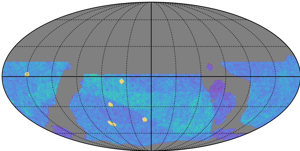
weather_cloudso6v3.4_10yrs WFD z band: NVisits
