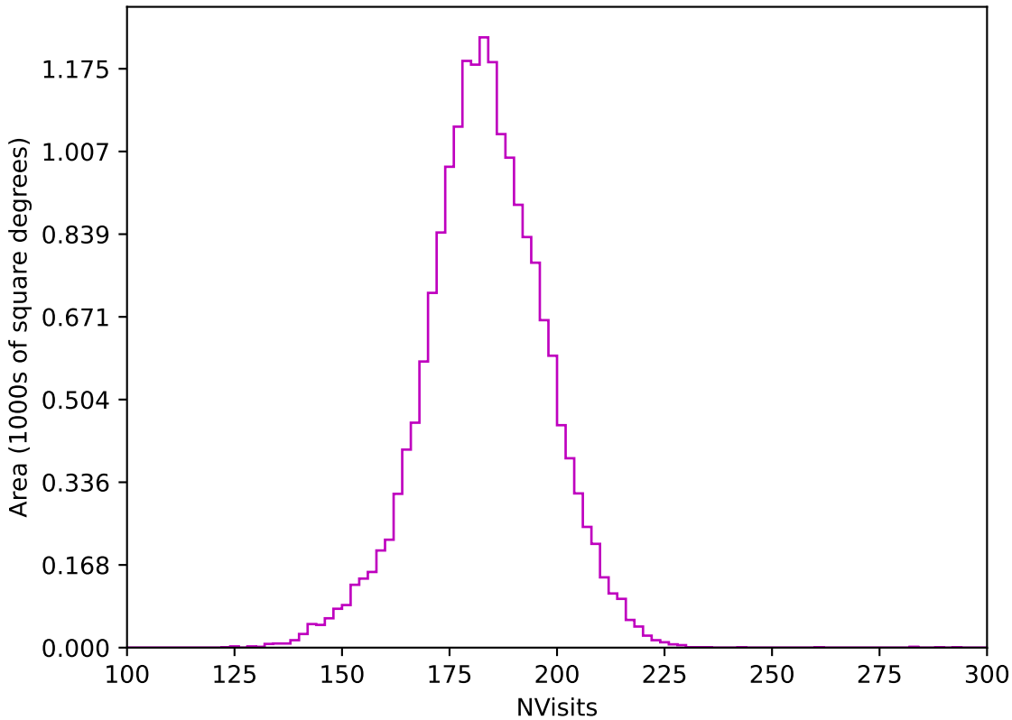
weather_cloudso6v3.4_10yrs WFD z band: NVisits
