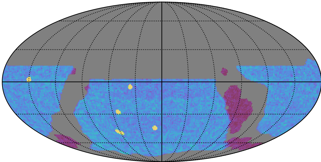
weather_cloudso6v3.4_10yrs WFD y band: NVisits
