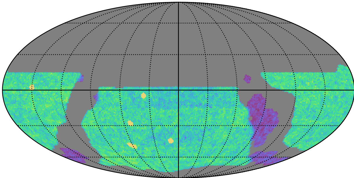
weather_cloudso6v3.4_10yrs WFD u band: NVisits
