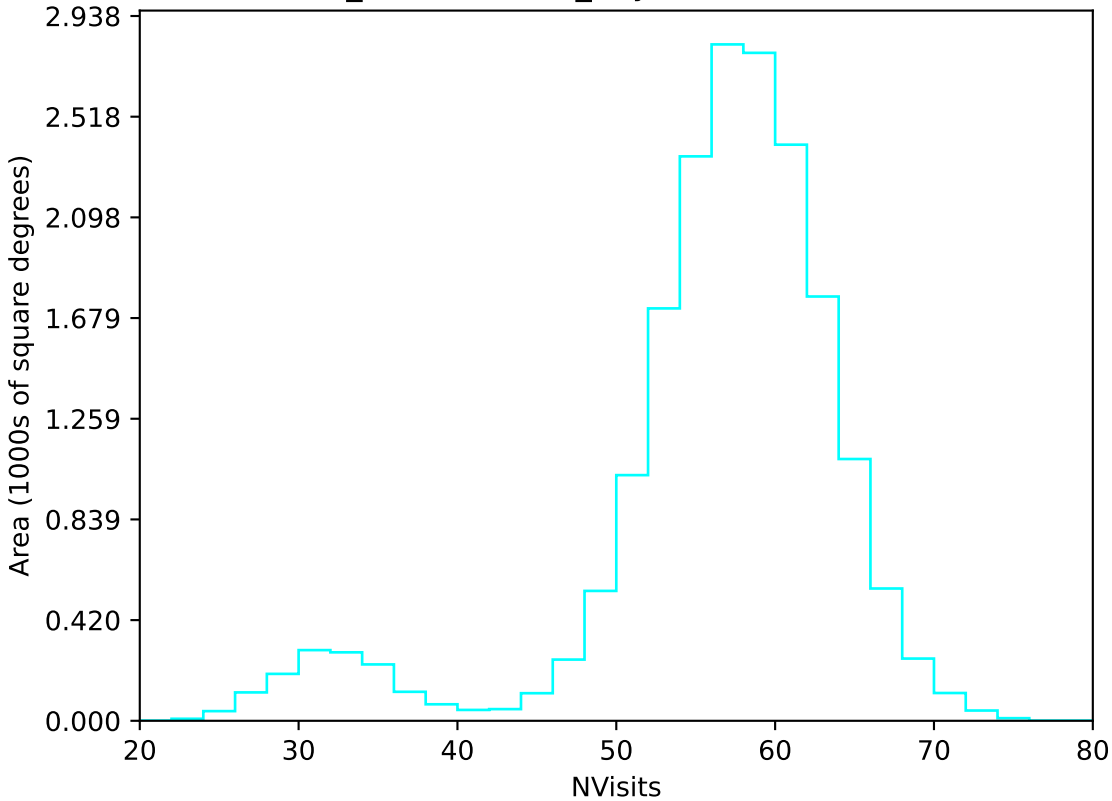
weather_cloudso6v3.4_10yrs WFD u band: NVisits
