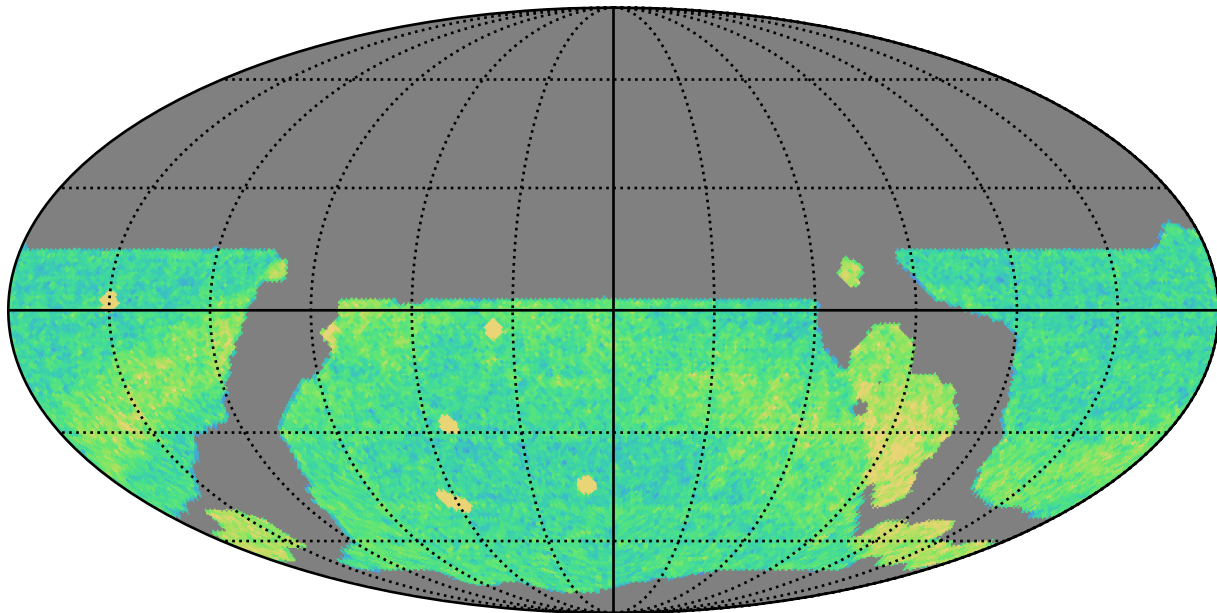
weather_cloudso6v3.4_10yrs WFD r band: NVisits
