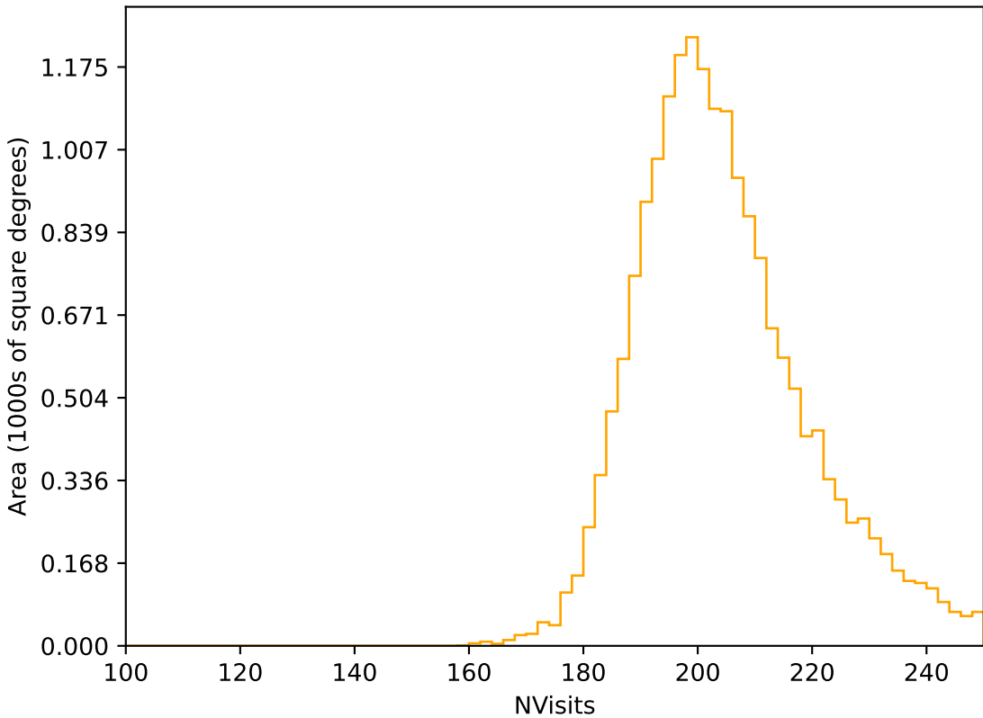
weather_cloudso6v3.4_10yrs WFD r band: NVisits
