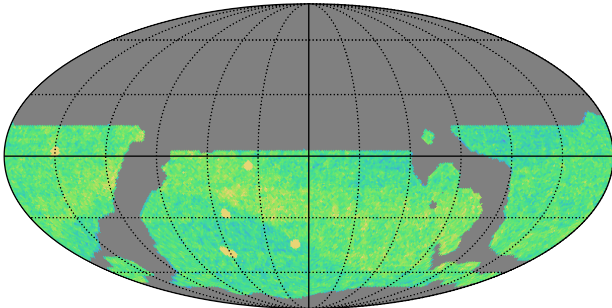
weather_cloudso6v3.4_10yrs WFD i band: NVisits
