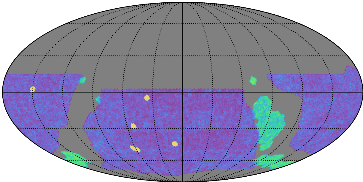
weather_cloudso6v3.4_10yrs WFD g band: NVisits
