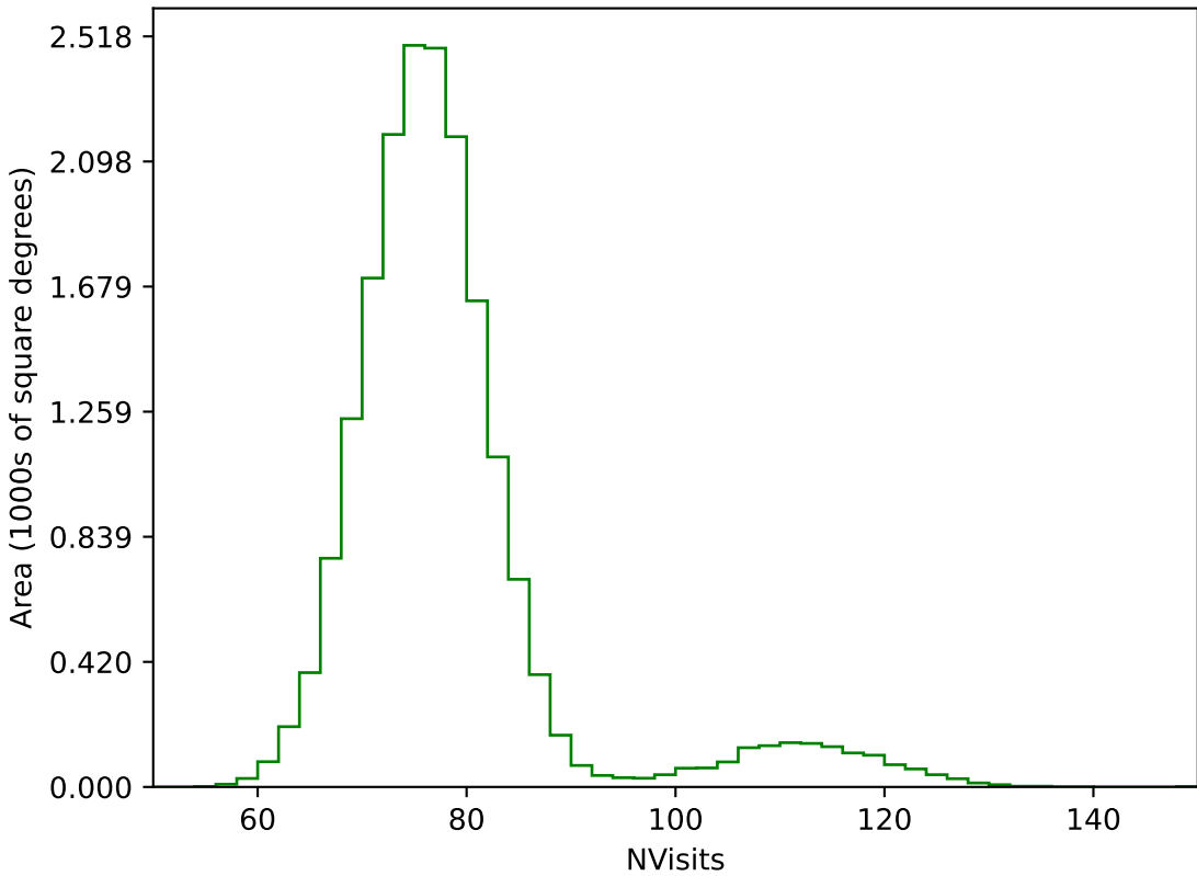
weather_cloudso6v3.4_10yrs WFD g band: NVisits
