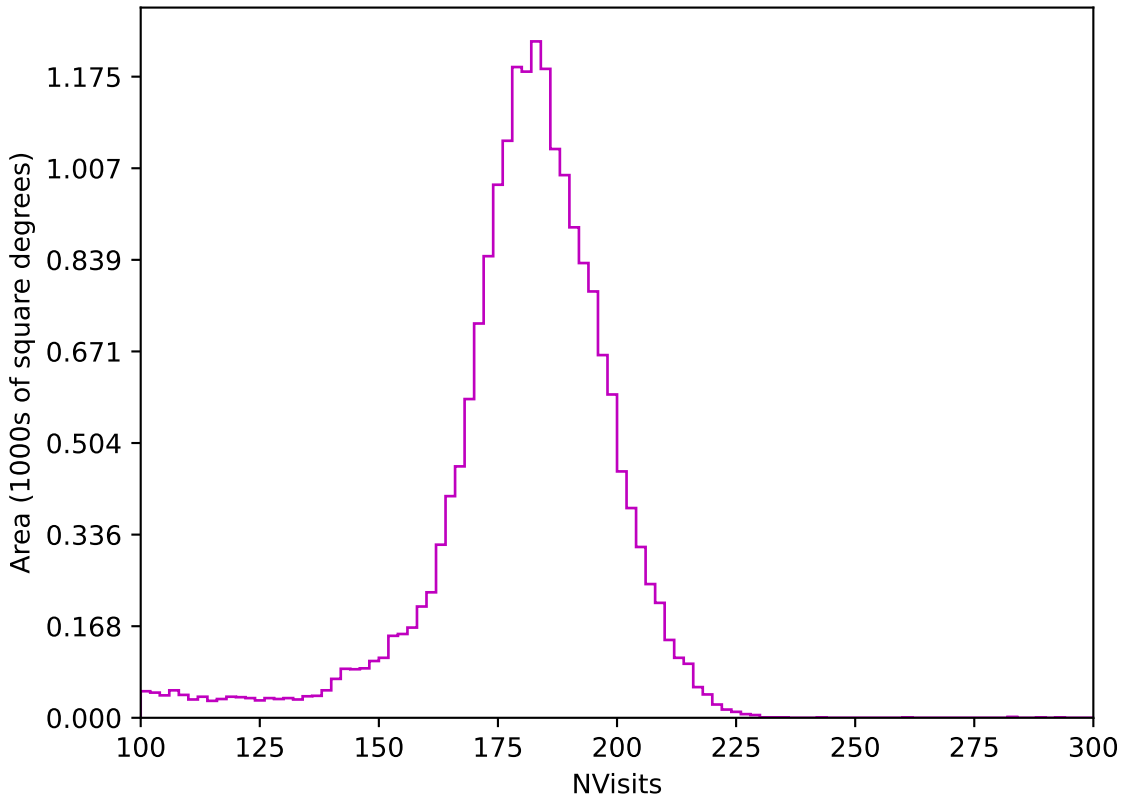
weather_cloudso6v3.4_10yrs All sky z band: NVisits
