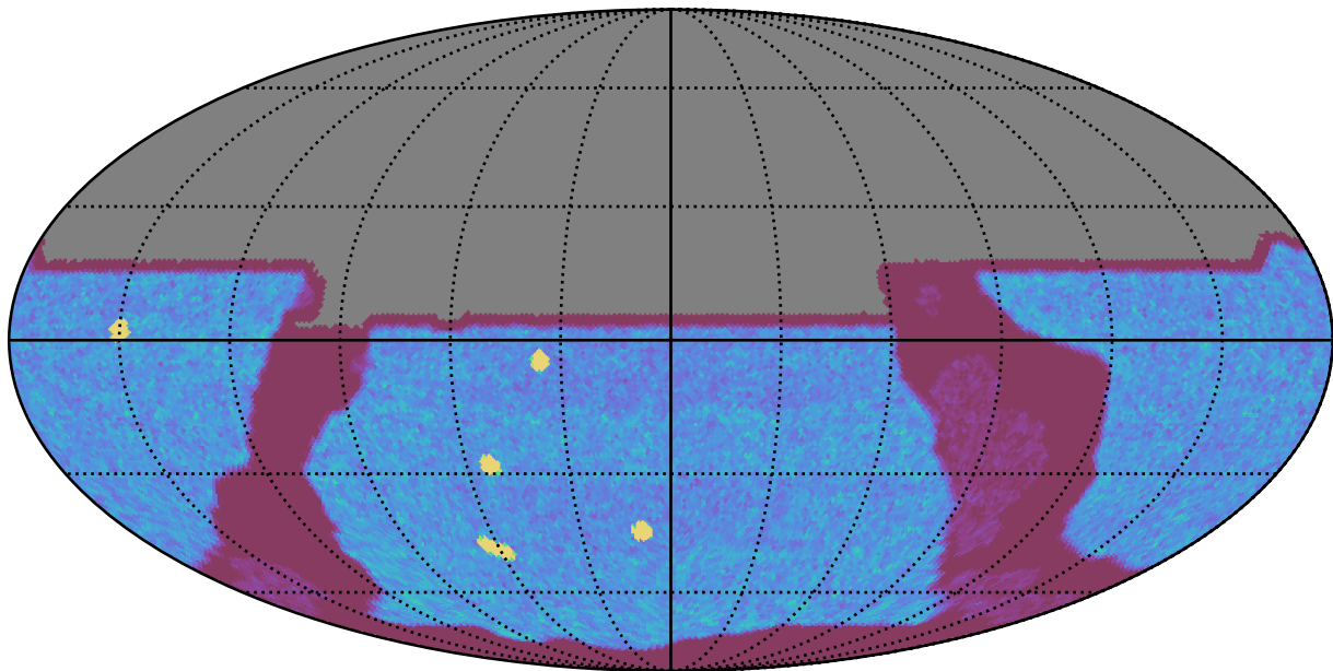
weather_cloudso6v3.4_10yrs All sky y band: NVisits
