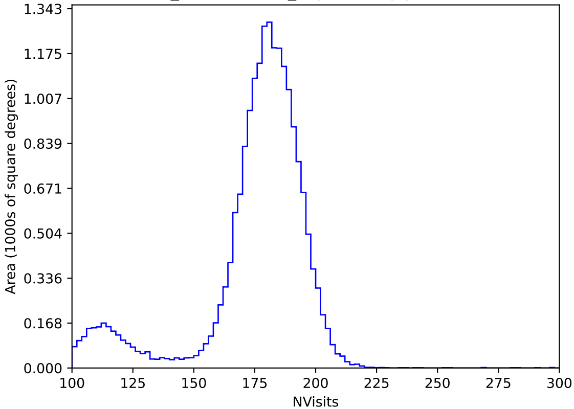
weather_cloudso6v3.4_10yrs All sky y band: NVisits
