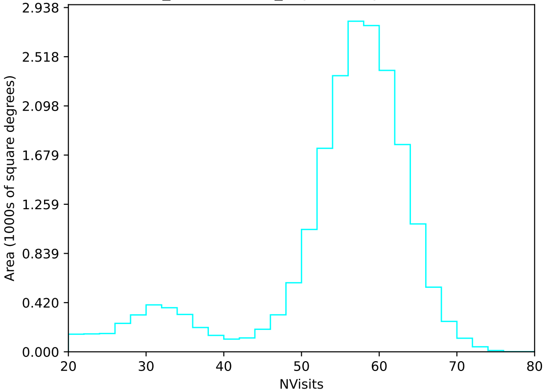
weather_cloudso6v3.4_10yrs All sky u band: NVisits
