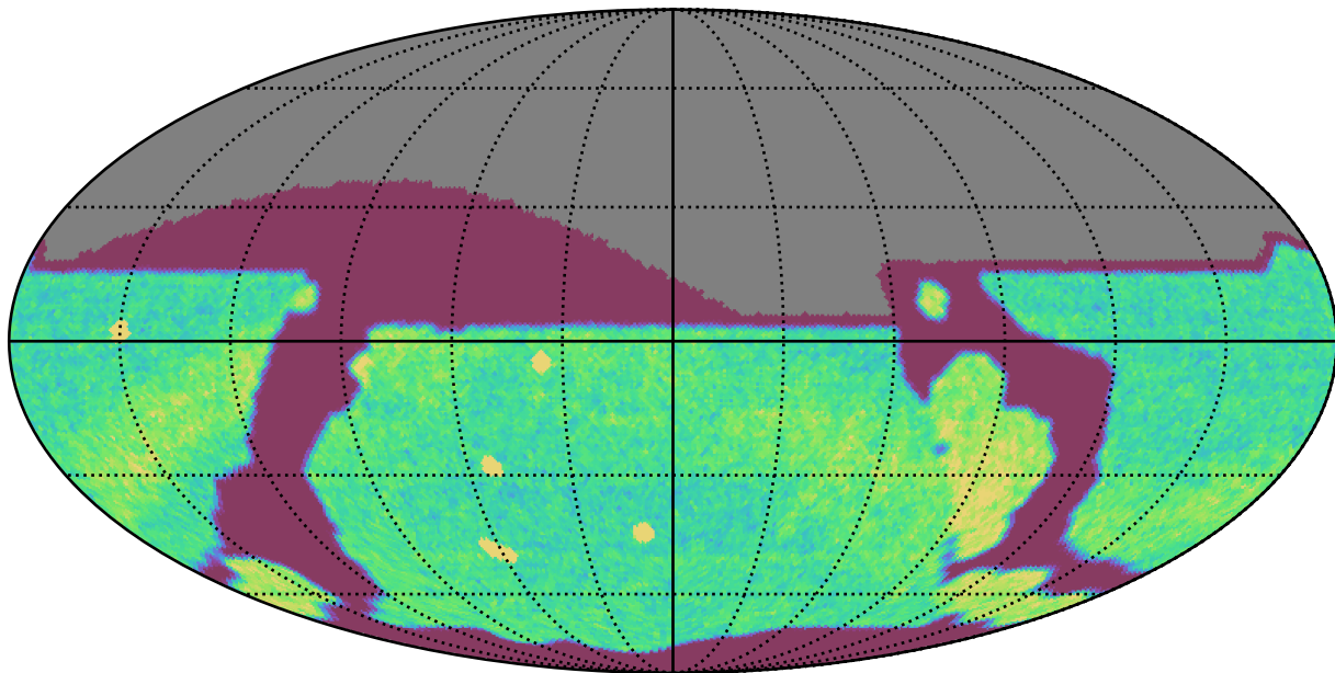
weather_cloudso6v3.4_10yrs All sky r band: NVisits
