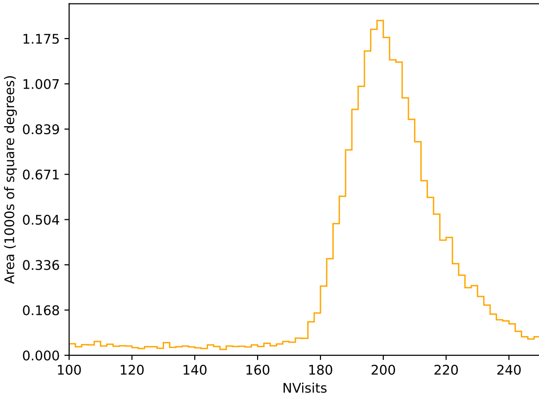
weather_cloudso6v3.4_10yrs All sky r band: NVisits
