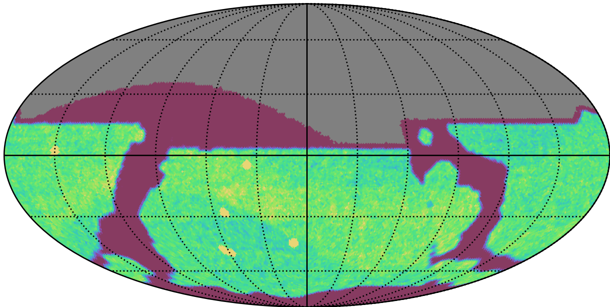
weather_cloudso6v3.4_10yrs All sky i band: NVisits
