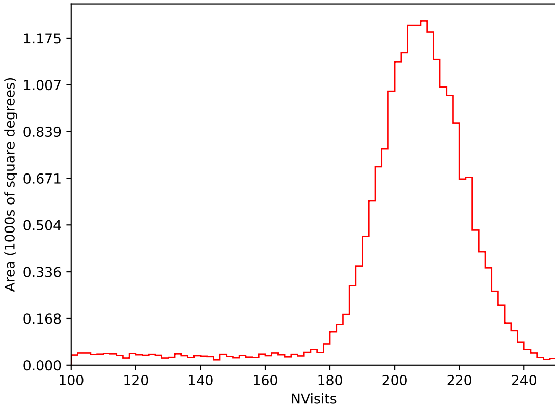
weather_cloudso6v3.4_10yrs All sky i band: NVisits
