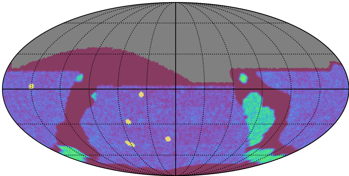
weather_cloudso6v3.4_10yrs All sky g band: NVisits
