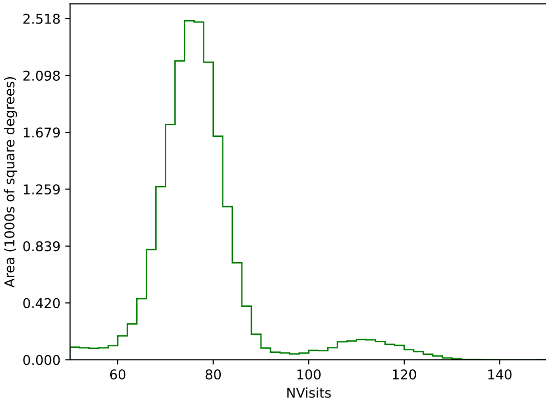
weather_cloudso6v3.4_10yrs All sky g band: NVisits
