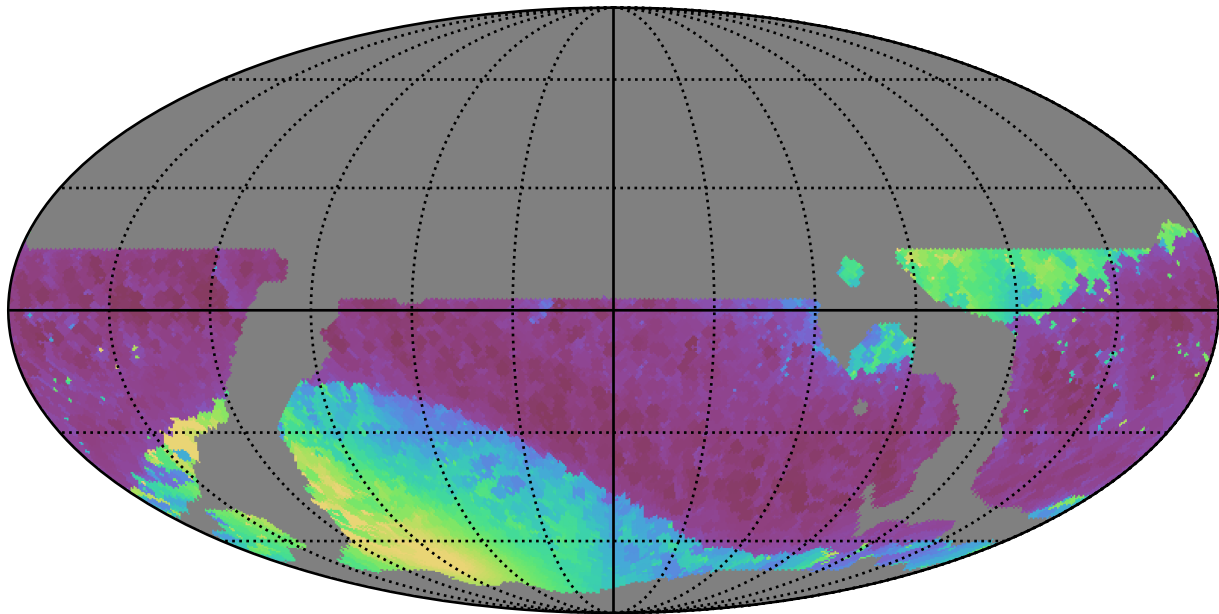
weather_cloudso6v3.4_10yrs WFD z band: Min solarElong
