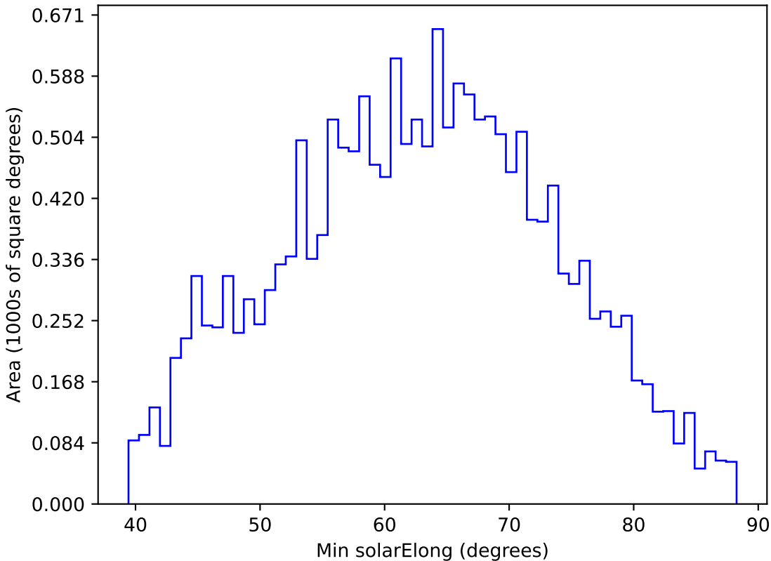
weather_cloudso6v3.4_10yrs WFD y band: Min solarElong
