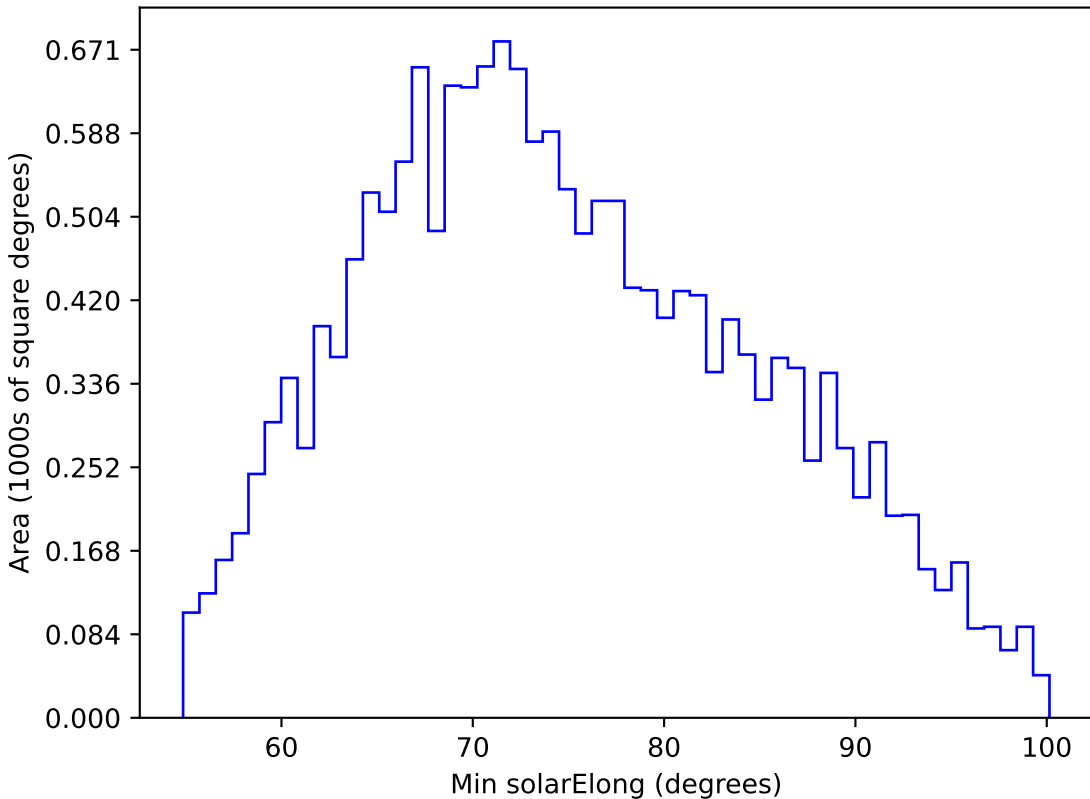
weather_cloudso6v3.4_10yrs WFD u band: Min solarElong
