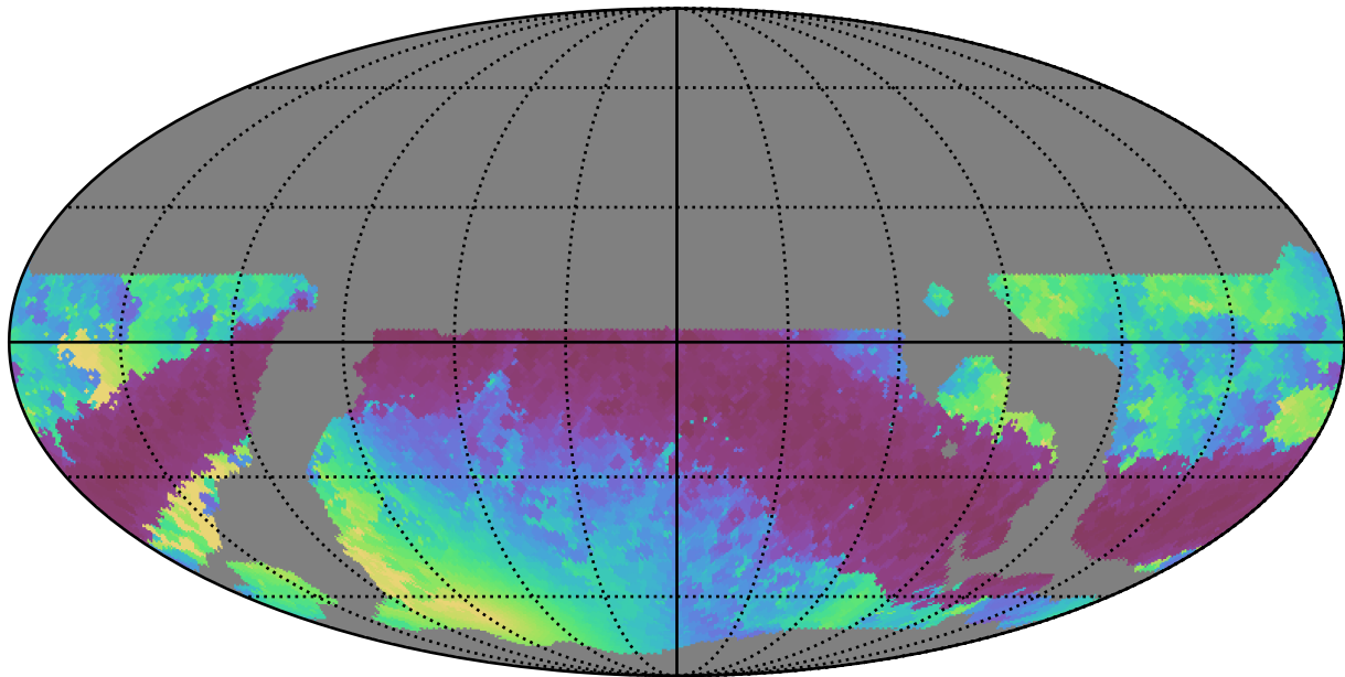
weather_cloudso6v3.4_10yrs WFD r band: Min solarElong
